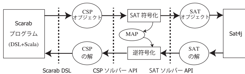
図 1. Scarab の構成
